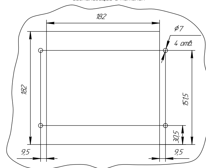
Разметка под крепление блока сигнализации и питания
